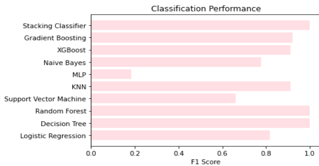
Fig 15 F1 Score graph
